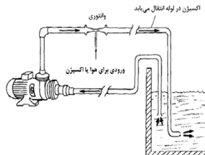
شکل ۱۷. هواده جت حلقوی «Fixed-Head»
