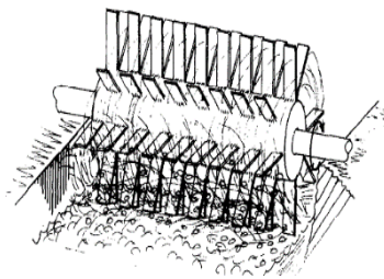
شکل ۹. هواده سطحی با محور افقی با تیغه‌های شعاعی مأخذ: (Cumby, 1987)
