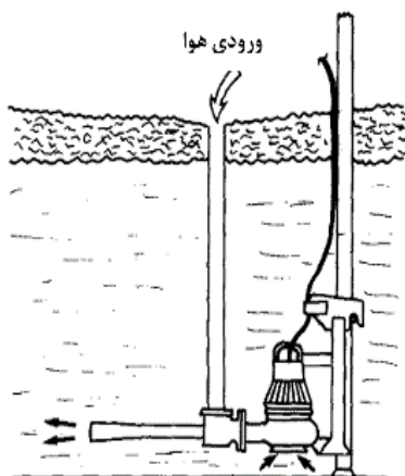
شکل ۱۸. هواده «ویتوکس»
