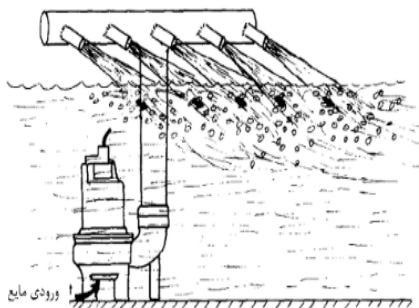
شکل ۱۵. هواده «Jet-Aero-Mix» مأخذ: (Cumby, 1987)
