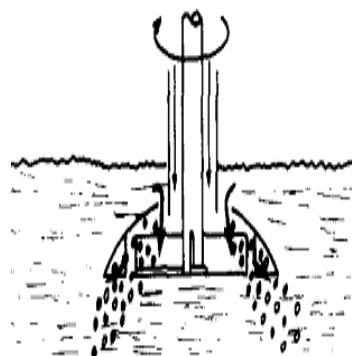
شکل ۱۱. پیشران با تیغه های خم کن محیطی ثابت
