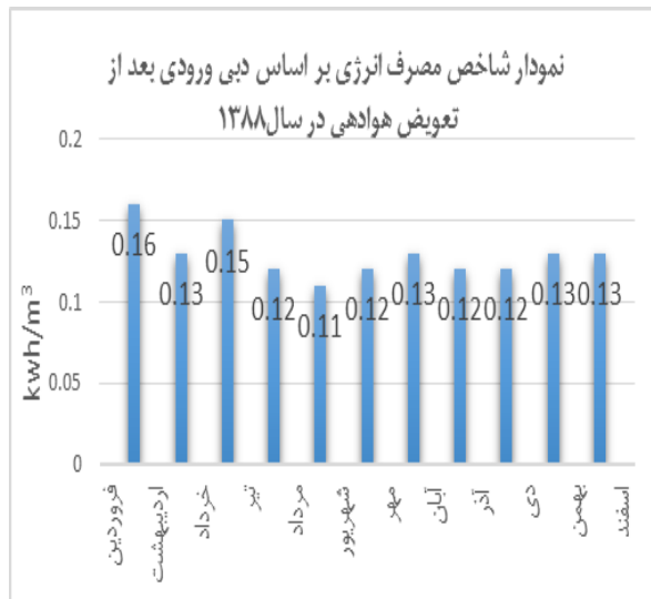
نمودار ۳. نمودار شاخص مصرف انرژی بر اساس دبی ورودی بعد از تعویض هوادهی در سال ۱۳۸۸ مأخذ: (Sadeghi et al., 2011)
