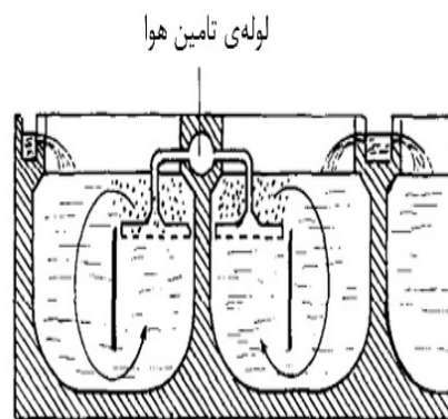
شکل ۴. هوادهای عمودی برای بهبود سیرکولاسیون، و افزایش نگر داشت حباب (سیستم اینکا) ۱ مأخذ: (Cumby, 1987)
