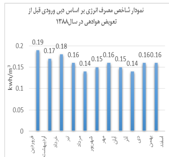
نمودار ۲. نمودار شاخص مصرف انرژی بر اساس دبی ورودی
