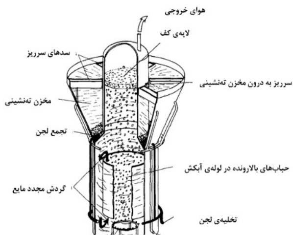
شکل ۶. «بیوهوک راکتور» برای پسماند صنعتی
