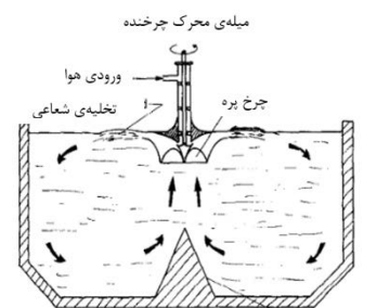
پروفل مخزن برای افزایش گردش
