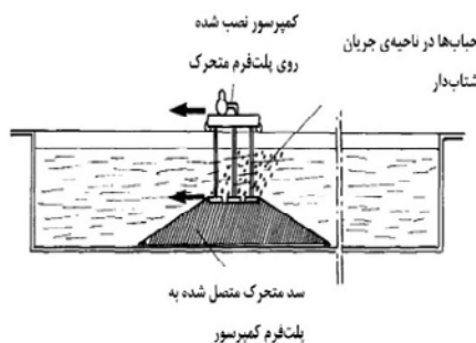
شکل ۳. هواده با نازل‌های متحرک برای افزایش نگه داشت حباب (سیستم دنجس) مأخذ: (Cumby, 1987)
