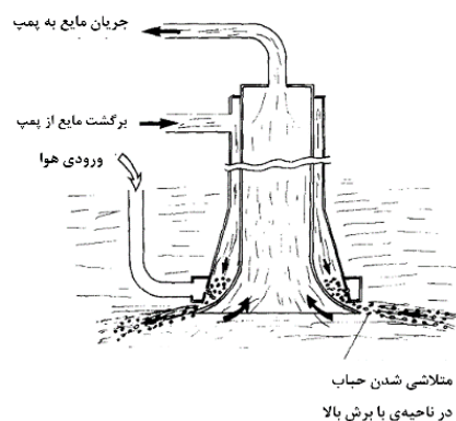
شکل ۱۶. هواده ایجکتور
