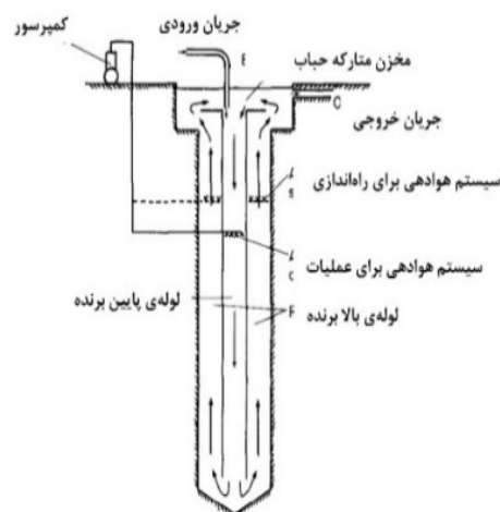
شکل ۵. سیستم تصفیه پساب «دیپ شفت» مأخذ: (Cumby, 1987)
